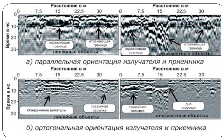
Рис. 2. Георадиолокационные записи, иллюстрирующие использование эффекта повышения разрешающей способности в полевых условиях за счет использования ортогонального расположения источника и приемника электромагнитных волн: а) при параллельном расположении излучателя и приемника; б) при ортогональном расположении излучателя и приемника [9]
